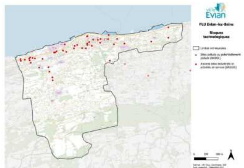
Carte 21 : Carte de la pollution des sols sur la commune d'Evian-les-Bains
