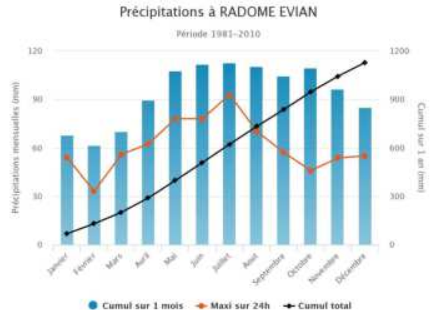
Graphique des précipitations sur la station d'Évian-les-Bains (source : Météo France)
